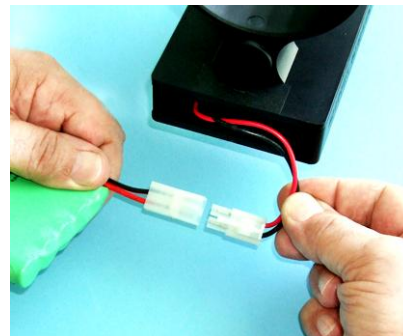
Presionar el gancho de seguridad para desbloquear el conector y desconectarlo
